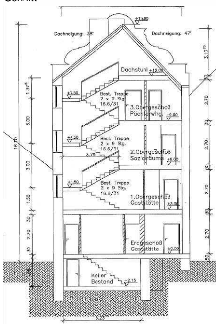
Schnitt
