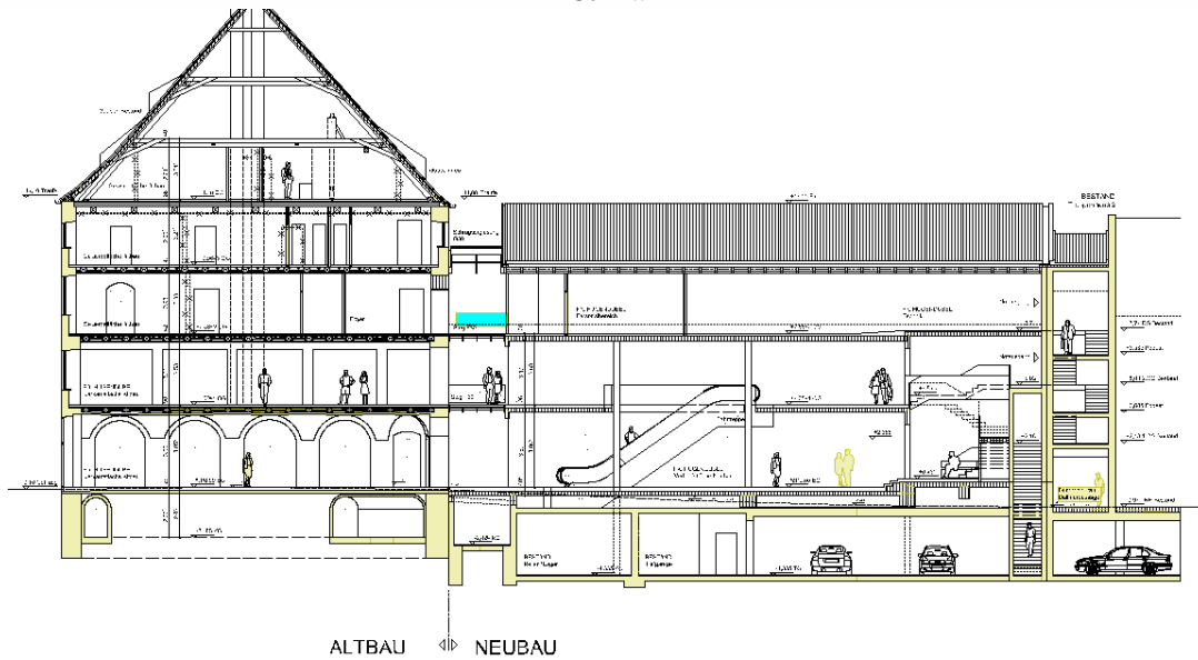
Längsschnitt B-B
